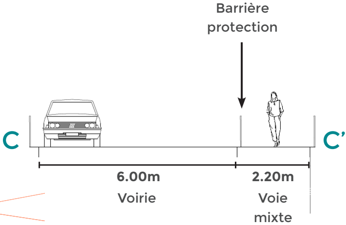
Traversée de la voie de chemin de fer
