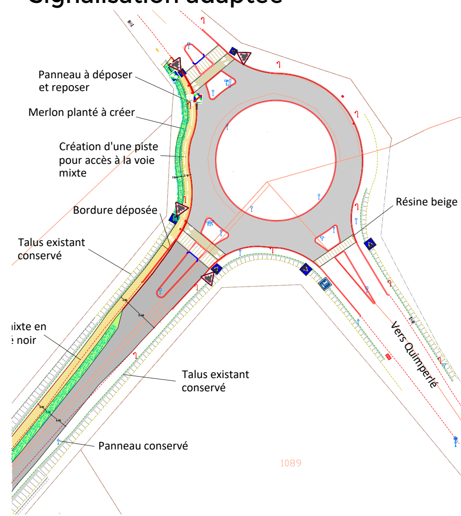
Aménagement Rond-point de Kergroës
