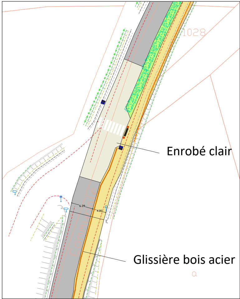
Traversée vers le centre équestre et GR
