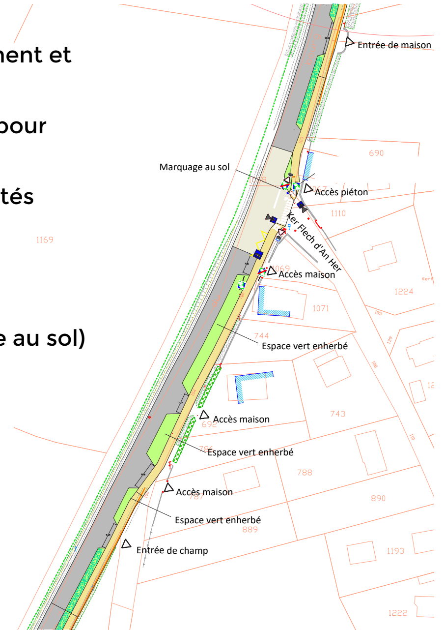
Carrefour de Kerflech d'An Her
